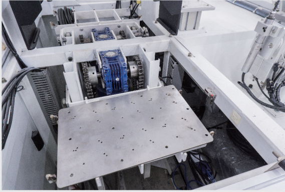
循環式供料機
