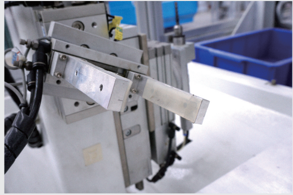
工件翻面台
